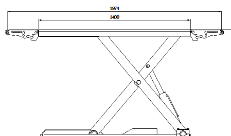
Dimensioni d'ingombro
